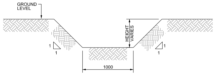
UNLINED DITCHES - D2
